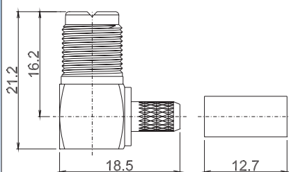
EMU-3802 MINI UHF JACK R/A CRIMP FOR CABLE - RG 58/U - RG 59/U - RG 6/U
